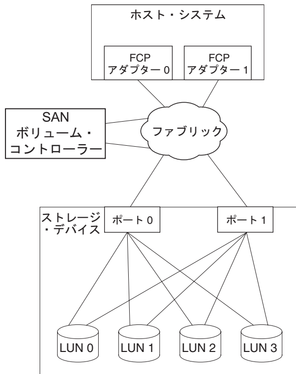
図2. ホスト・システムと SAN ボリューム・コントローラーを備えたディスク・ストレージ間のマルチパス接続
