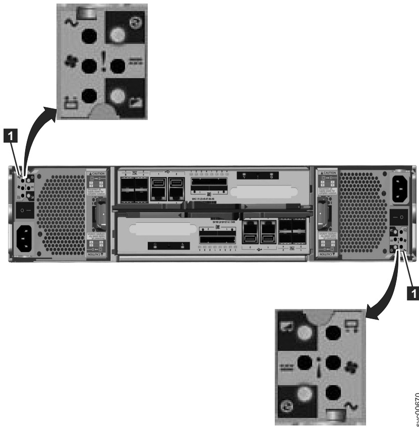
圖 18. 控制機箱電源供應器裝置上的 LED
