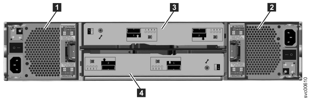
圖 6. 機型 2076-212 或機型 2076-224 擴充機箱的背面圖
