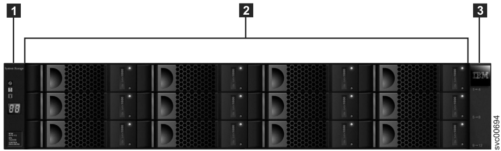
圖 2. 12 部磁碟機和兩個端蓋
