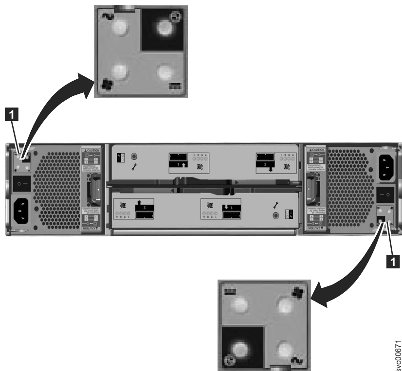
圖 17. 擴充機箱電源供應器裝置上的 LED
