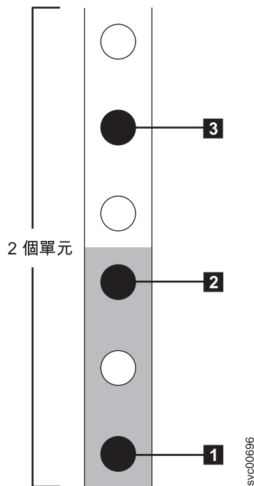
圖 9. 機架後方的孔位
