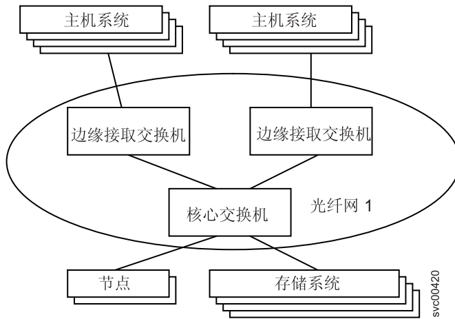
图 33. 采用中型光纤网的 SAN 配置
