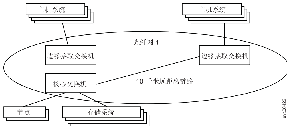
图 35. 跨两个站点的 SAN 配置
