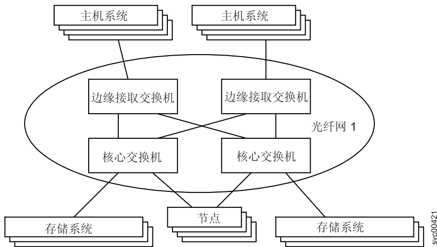
图 34. 采用大型光纤网的 SAN 配置
