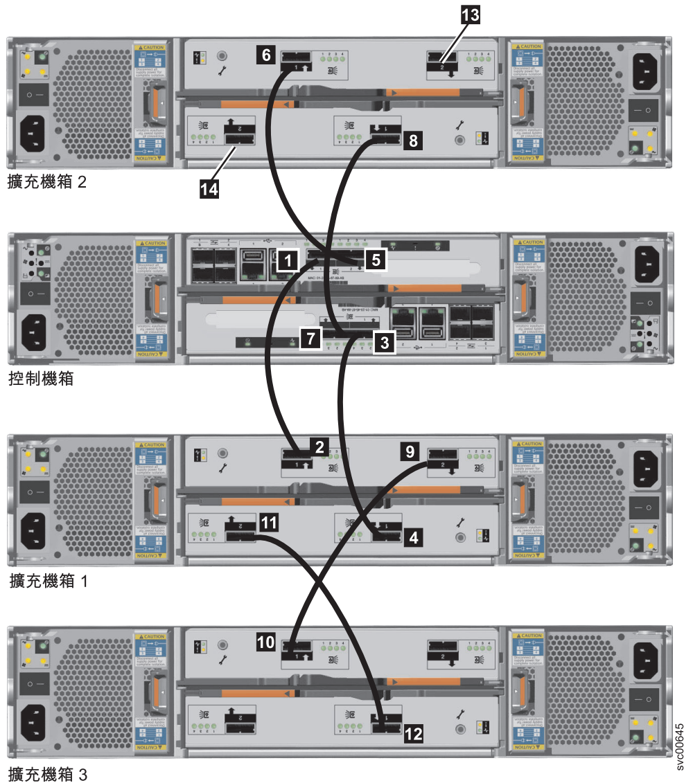
圖 12. 將 SAS 纜線連接至機箱
