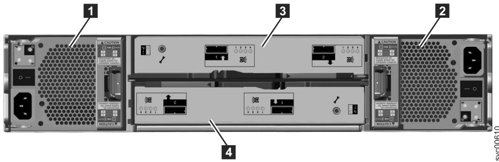
圖 6. 擴充機箱的背面圖
