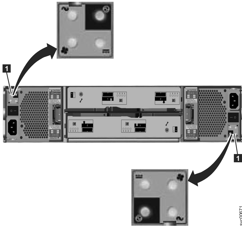
圖 13. 擴充機箱電源供應器單元上的 LED
