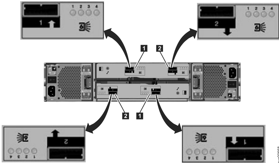
圖 7. 擴充機箱後方的 SAS 埠和 LED
