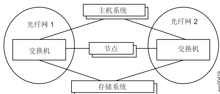
图 31. 简单 SAN 配置
