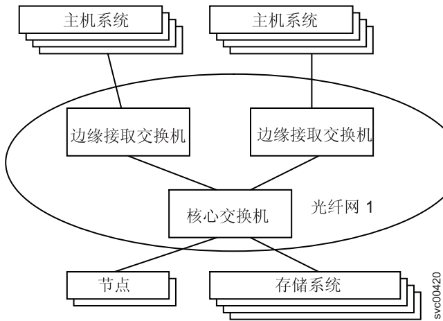
图 32. 采用中型光纤网的 SAN 配置
