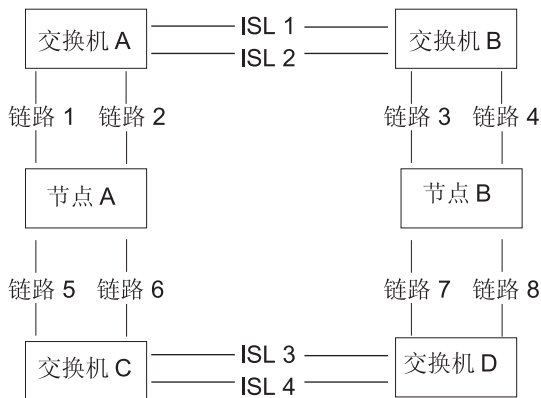
图 30. 在冗余配置中具有 ISL 的光纤网
