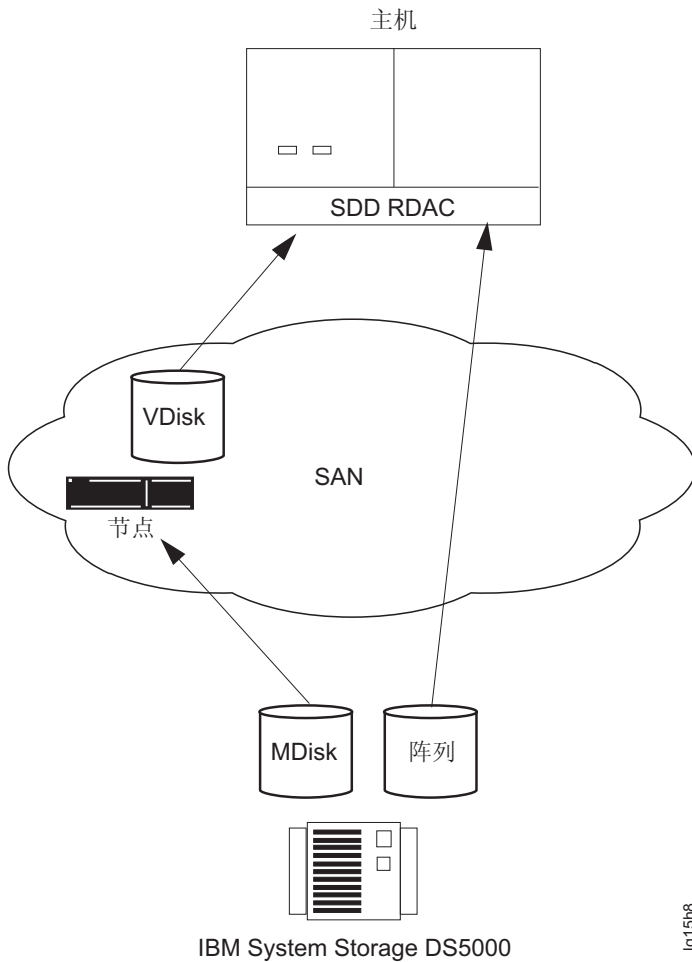
图 28. 一台主机上的 IBM DS5000 直接连接于与 SAN Volume Controller 节点
