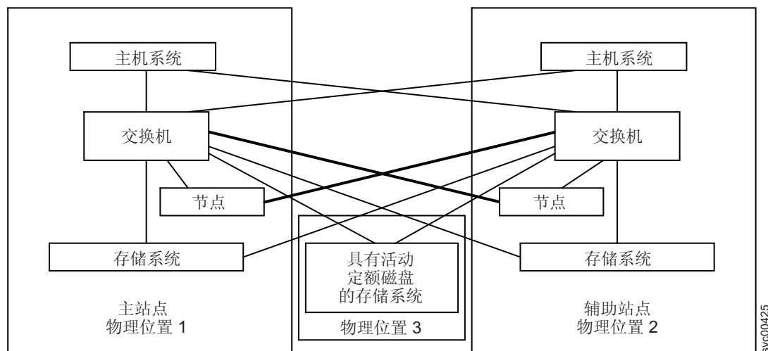
图 35. 定额磁盘位于第三个站点的拆分集群系统
