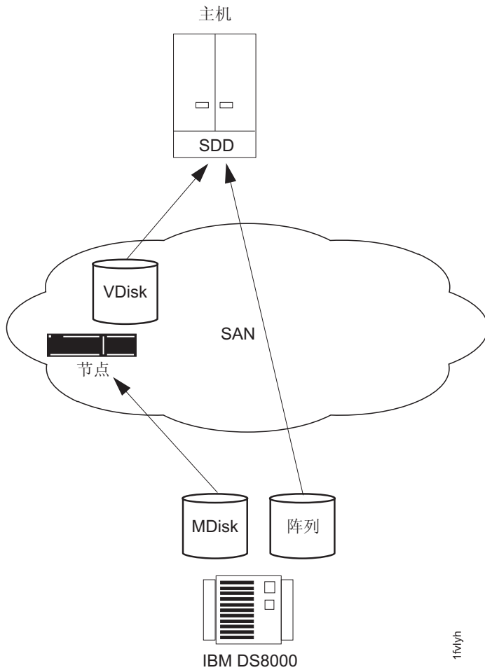
图 27. 使用 SAN Volume Controller 节点直接访问的 IBM System Storage DS8000 LU
