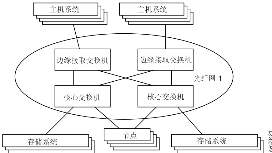
图 33. 采用大型光纤网的 SAN 配置
