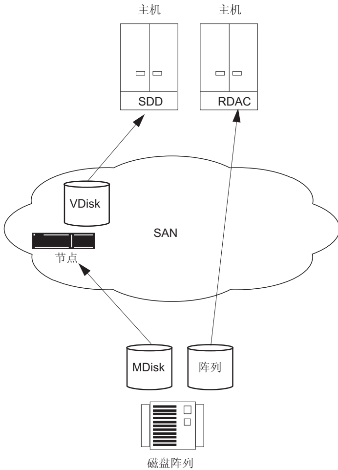
图 26. SAN Volume Controller 节点和主机间共享的存储系统
