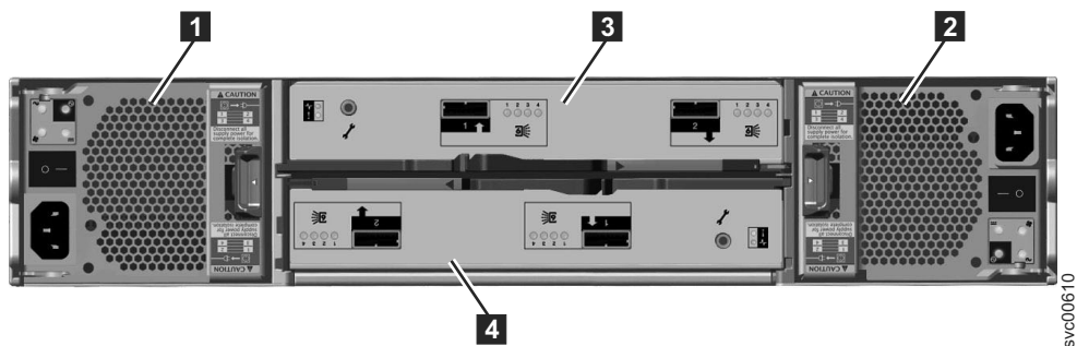
图 5. 扩展机柜的后视图
