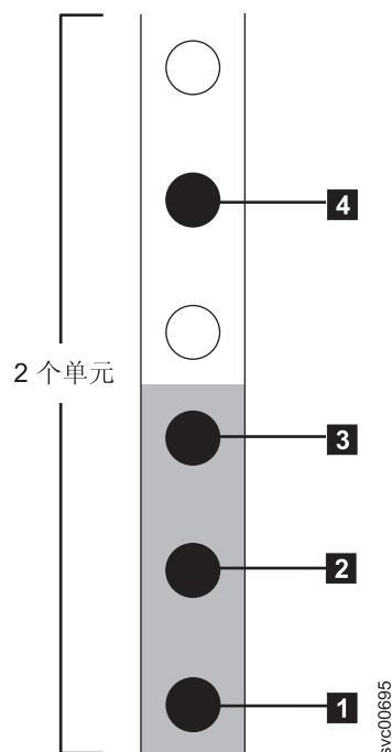
图 7. 机架前部的孔位置
