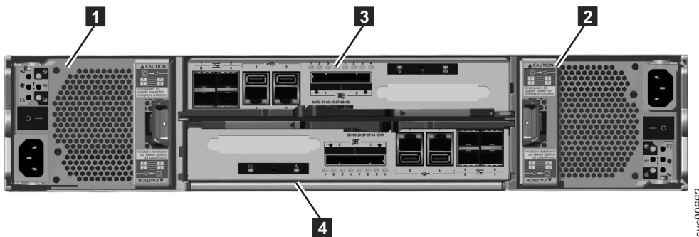
图 3. 控制机柜的后视图
