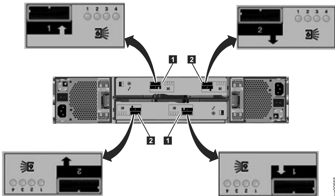
图 6. 扩展机柜后部的 SAS 端口和指示灯
