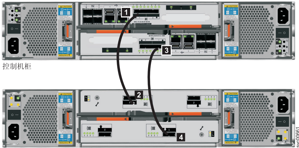
扩展机柜 1
