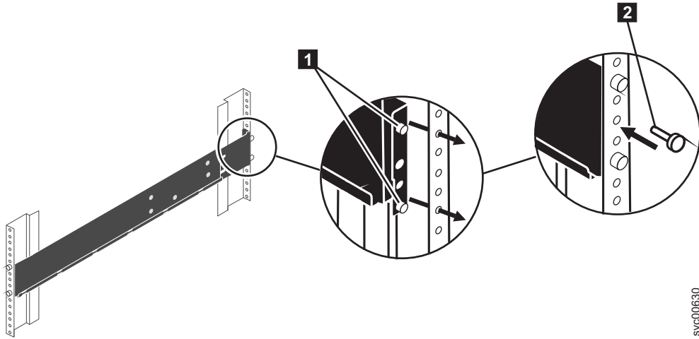
图 8. 将导轨组合件连接到机架式机箱
