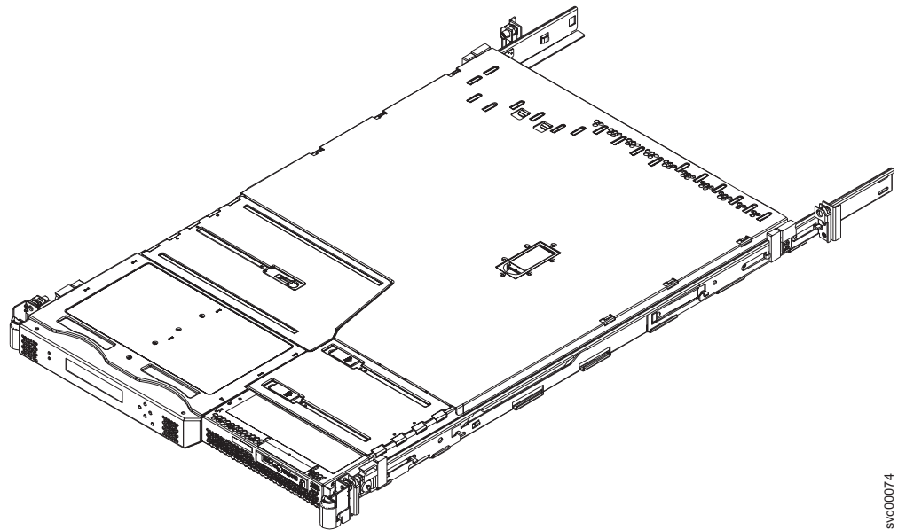
図3. SAN ボリューム・コントローラー 2145-8F2 ノード
