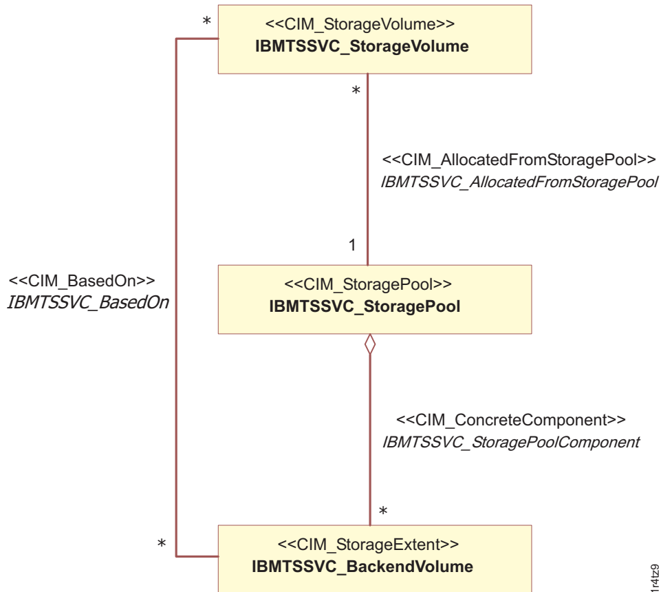
図7. SAN ボリューム・コントローラー用 CIM エージェントのエクステント・マッピング・サブプロファイルのハイレベルな概要
