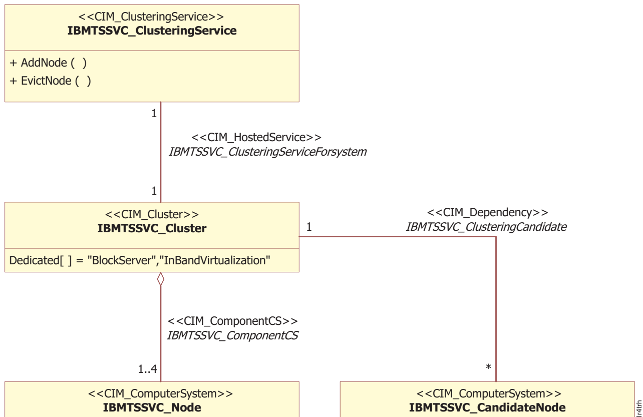
図 10. クラスタリング・インスタンスのクラス・ダイアグラム
