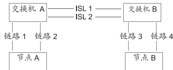
图 19. 在集群中节点之间使用交换机间链路的光纤网
