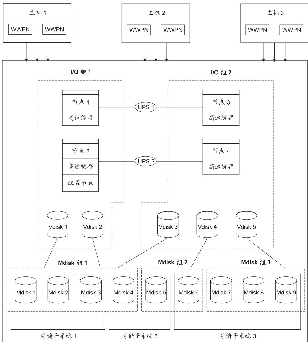
图 10. 虚拟化系统中的对象
