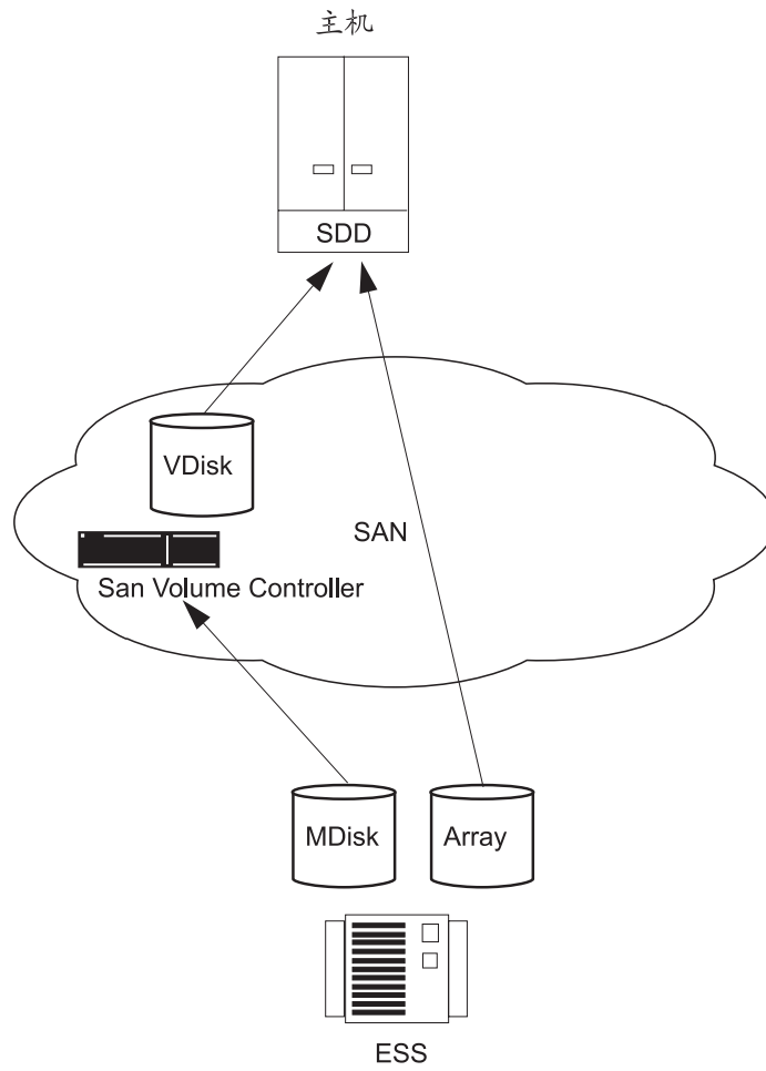
图 17. 使用 SAN Volume Controller 直接访问的 ESS LU
