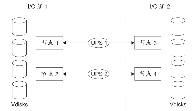
图 9. I/O 组和不间断电源部件之间的关系
