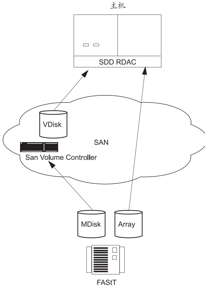
图 18. FASTT 使用一个主机上的 SAN Volume Controller 直接连接
