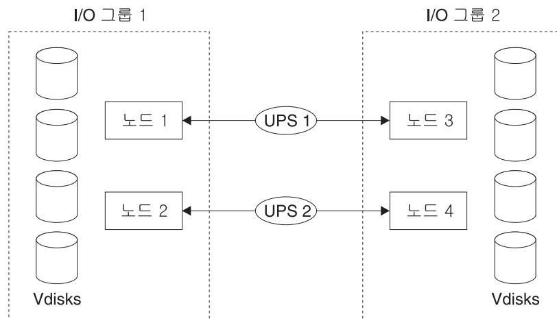
그림 9. I/O 그룹 및 무정전 전원 공급 장치 관계
