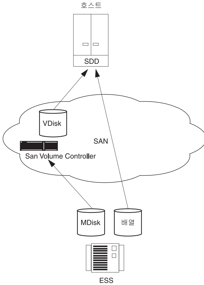
그림 17. 직접 및 SAN Volume Controller를 통해 액세스되는 ESS LU
